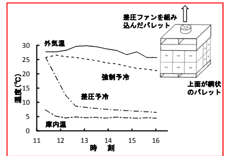
差圧予冷による品温変化と 現場での予冷装置の一例
